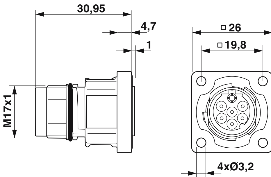
Rysunek wymiarowy
