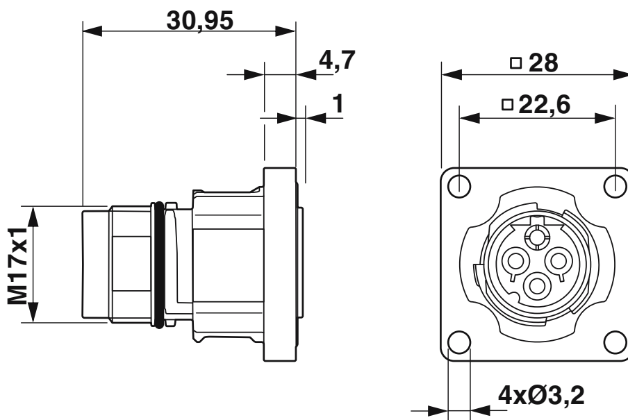
Rysunek wymiarowy
