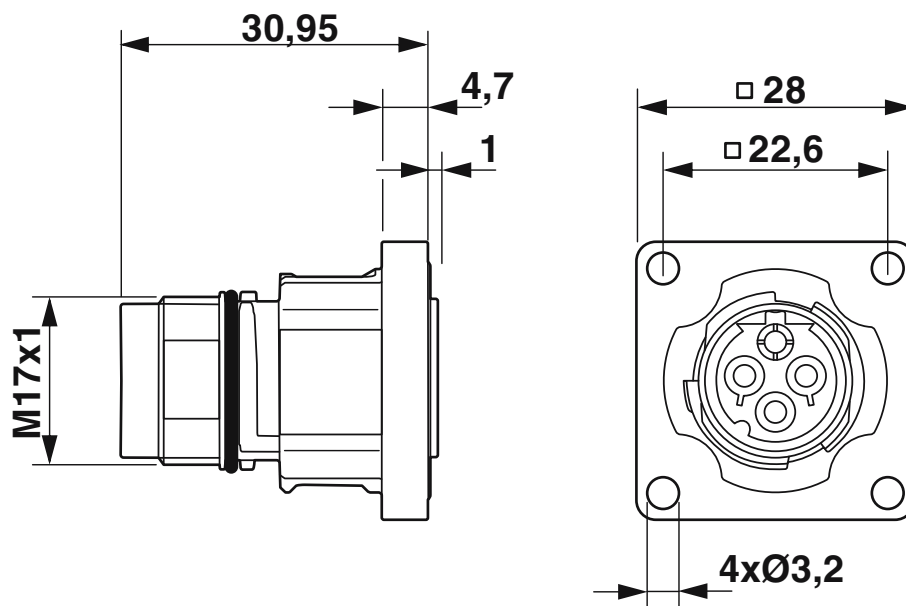
Rysunek wymiarowy
