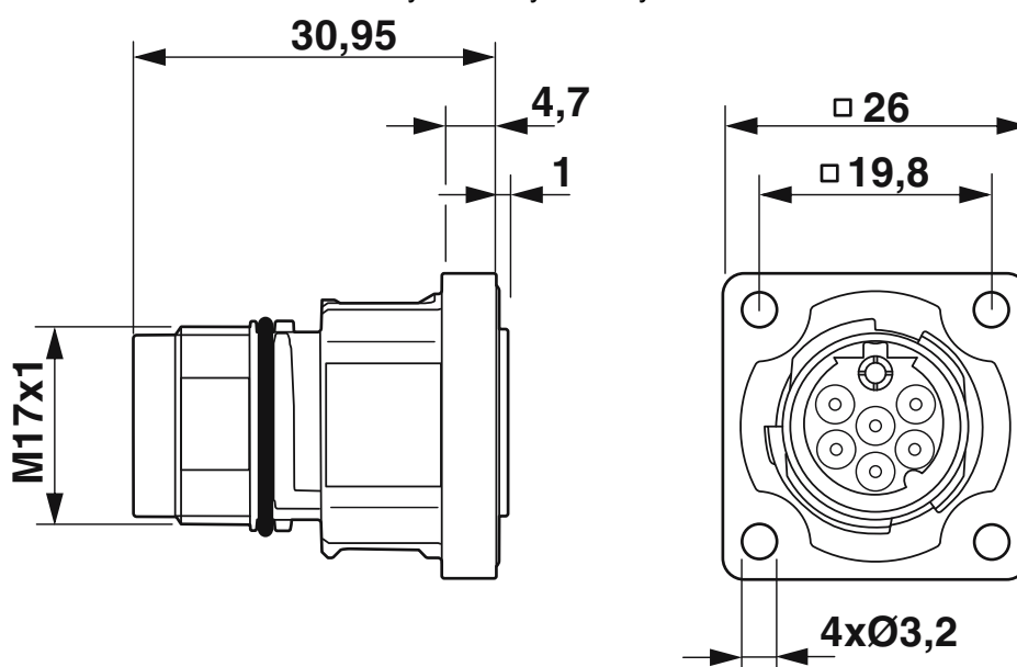
Rysunek wymiarowy
