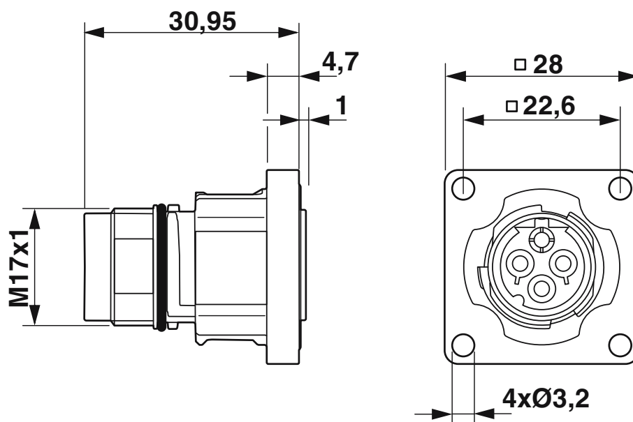
Rysunek wymiarowy
