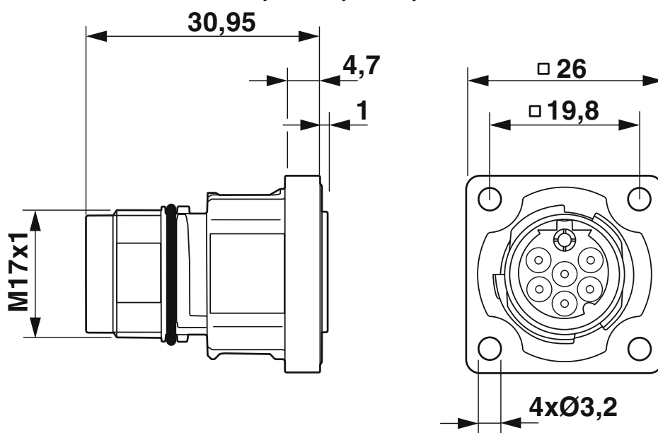
Rysunek wymiarowy
