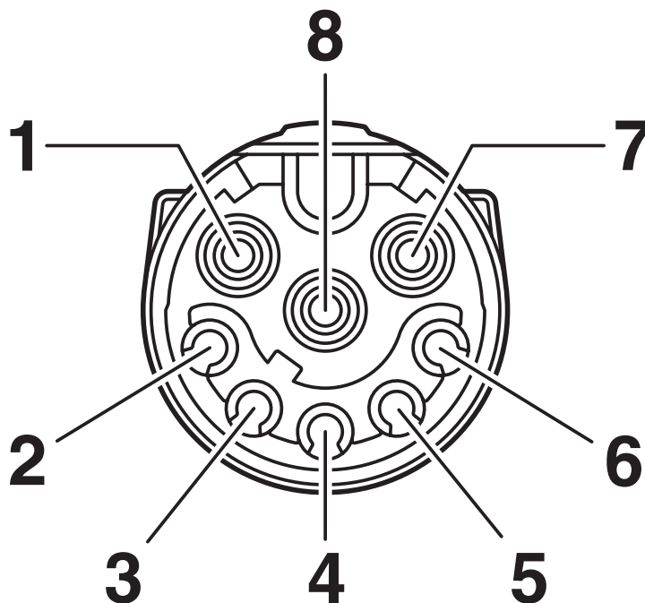
Rysunek schematyczny
