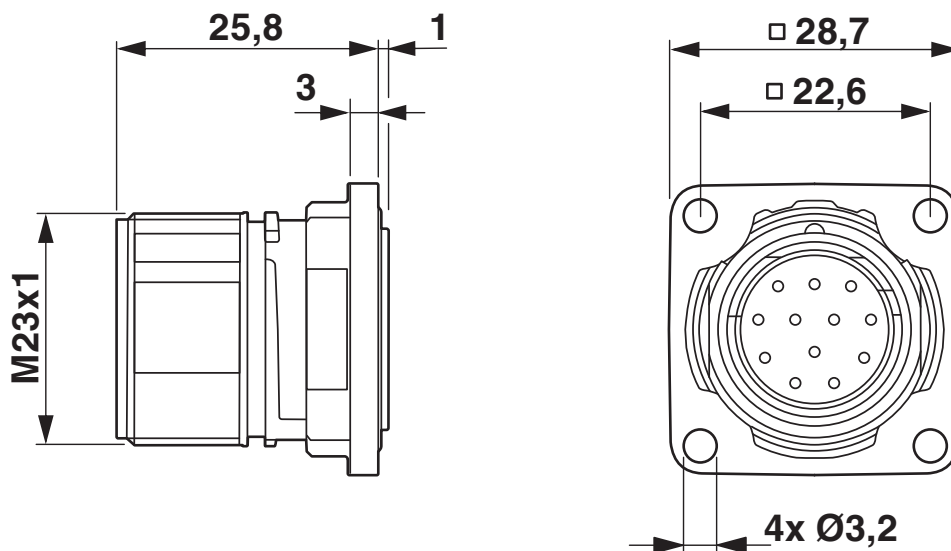
Rysunek wymiarowy
