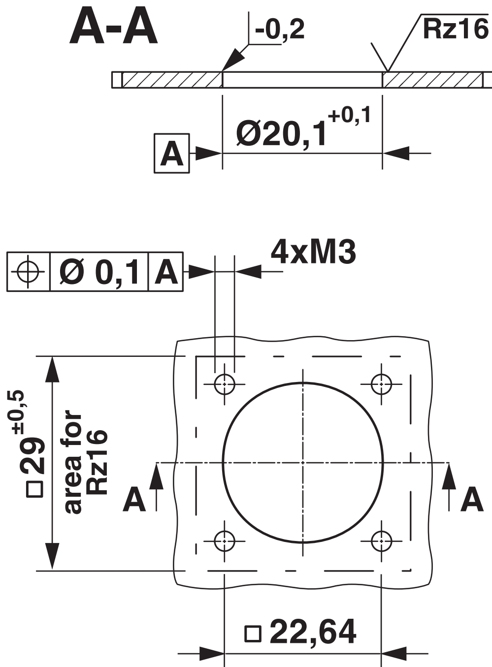
Rysunek wymiarowy
