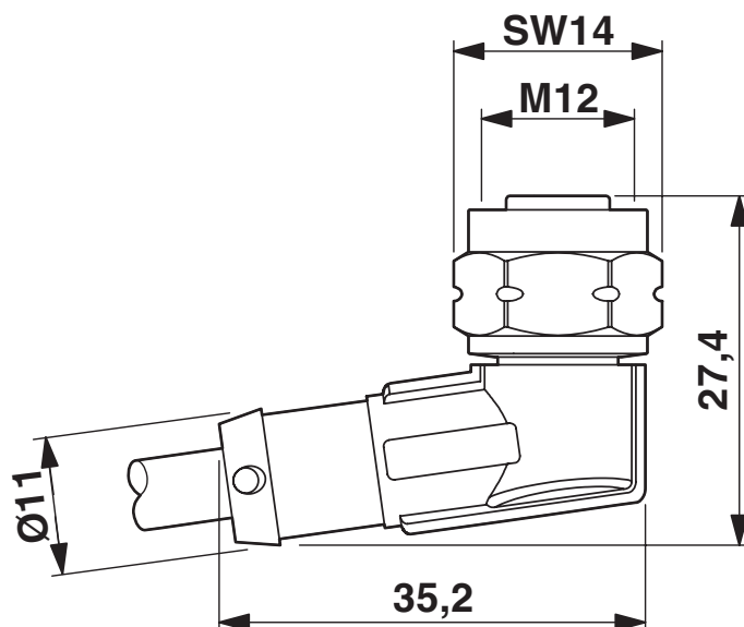
Rysunek wymiarowy
