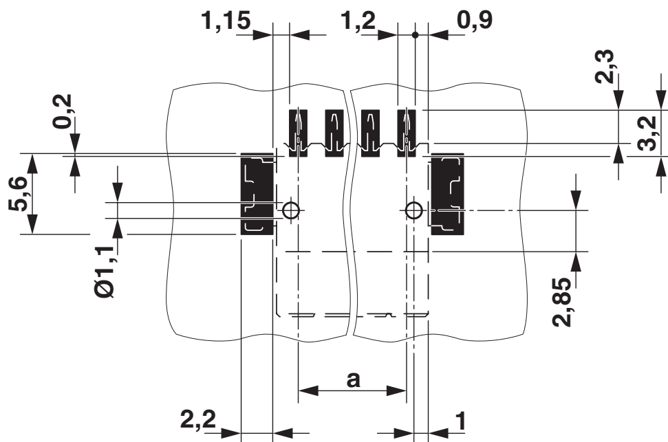
Otworowanie/geometria płytek lutowiczych
