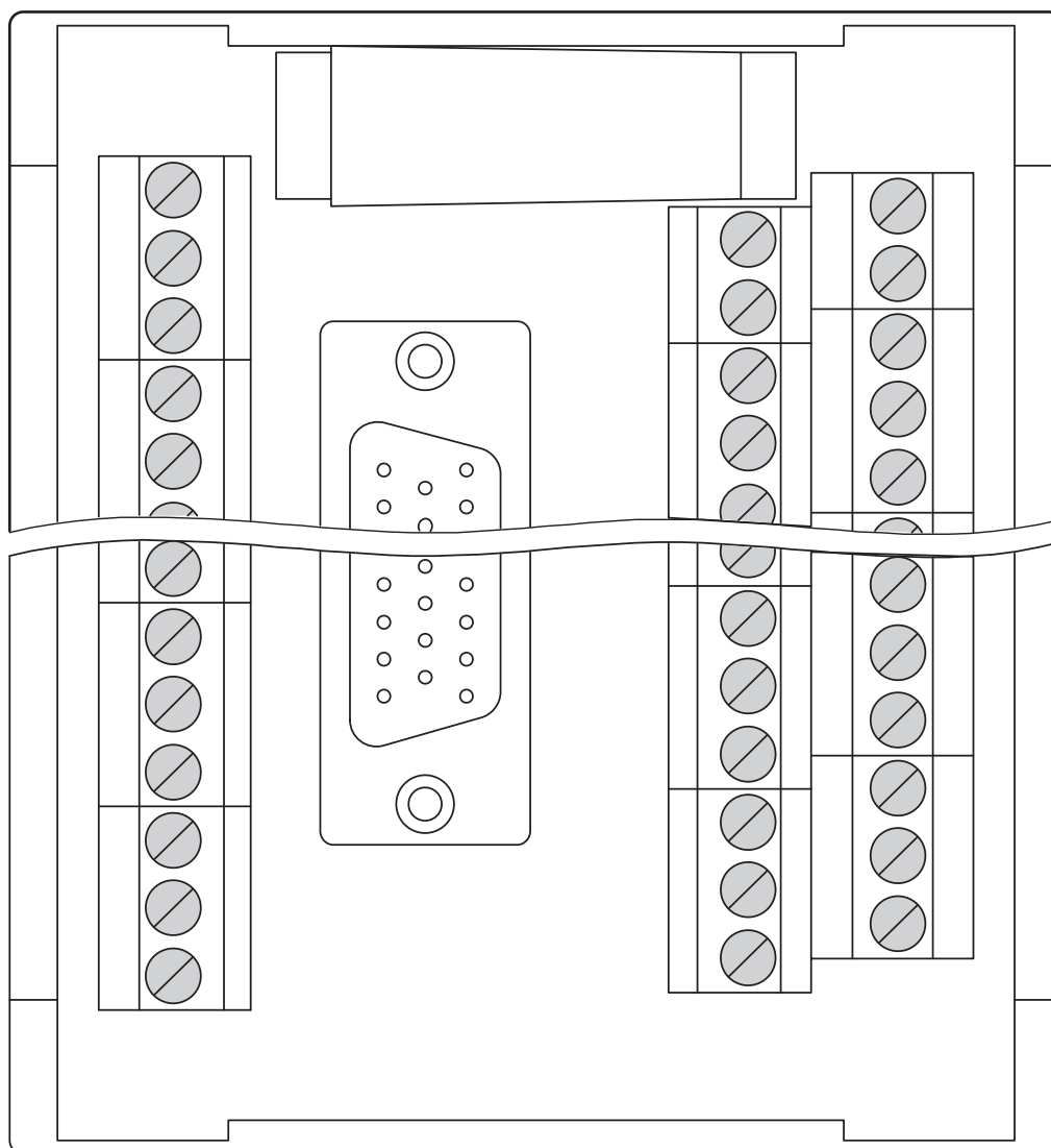
Rysunek schematyczny
