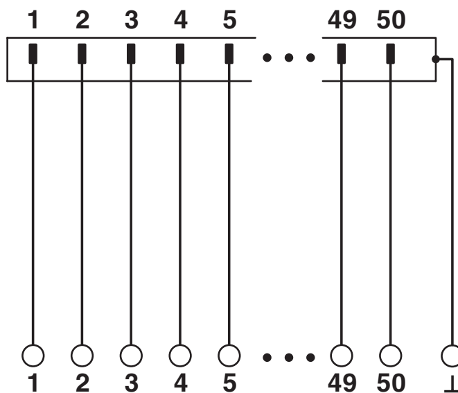
Schemat
