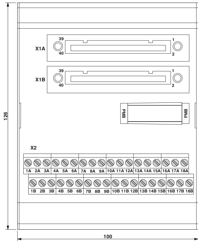
Rysunek wymiarowy
