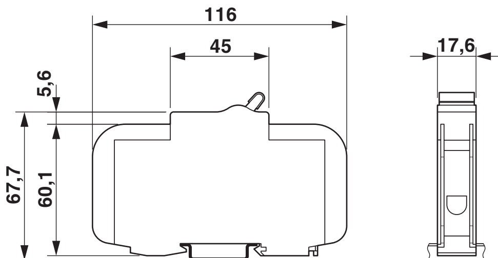
Rysunek wymiarowy
