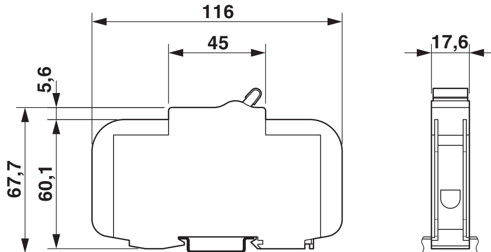
Rysunek wymiarowy
