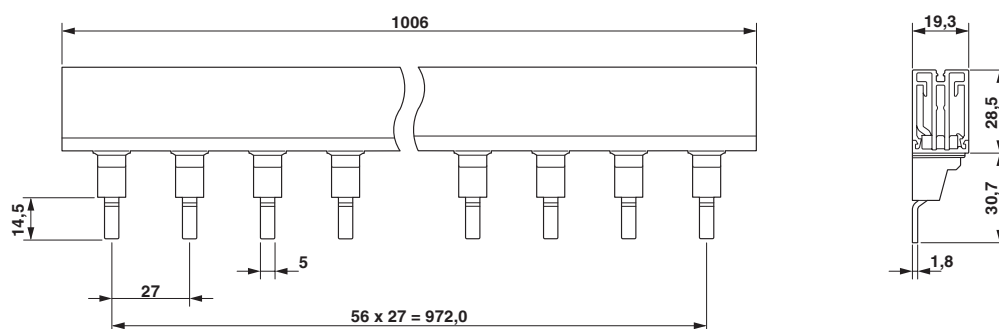
Rysunek wymiarowy
