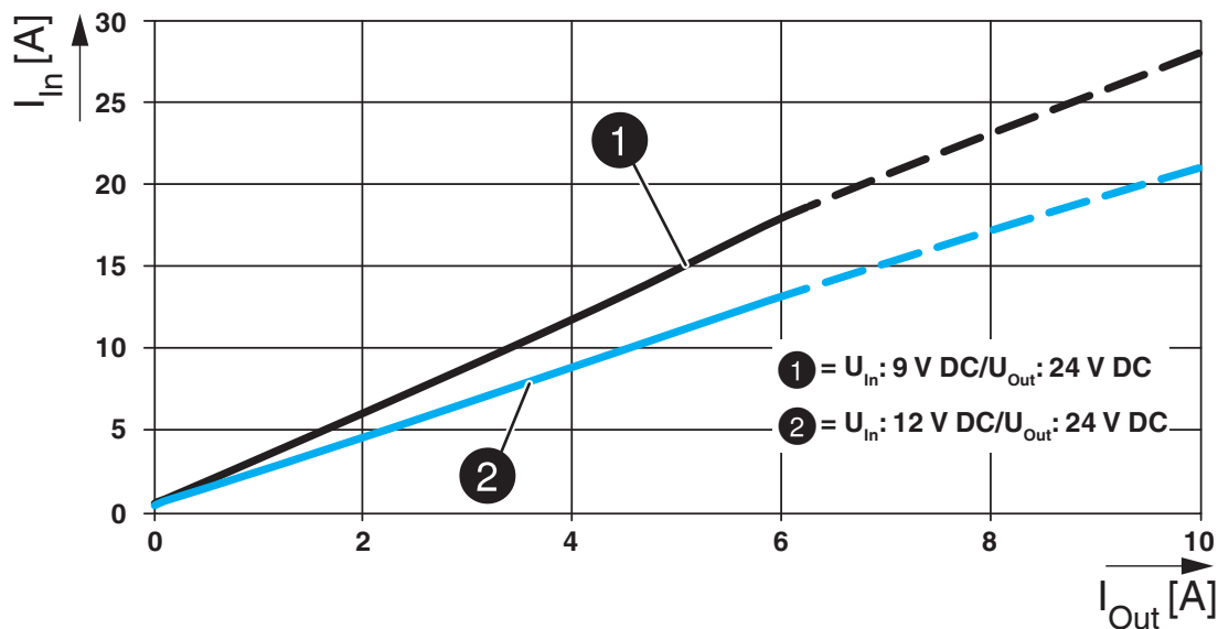
Prąd wejściowy/wyjściowy
