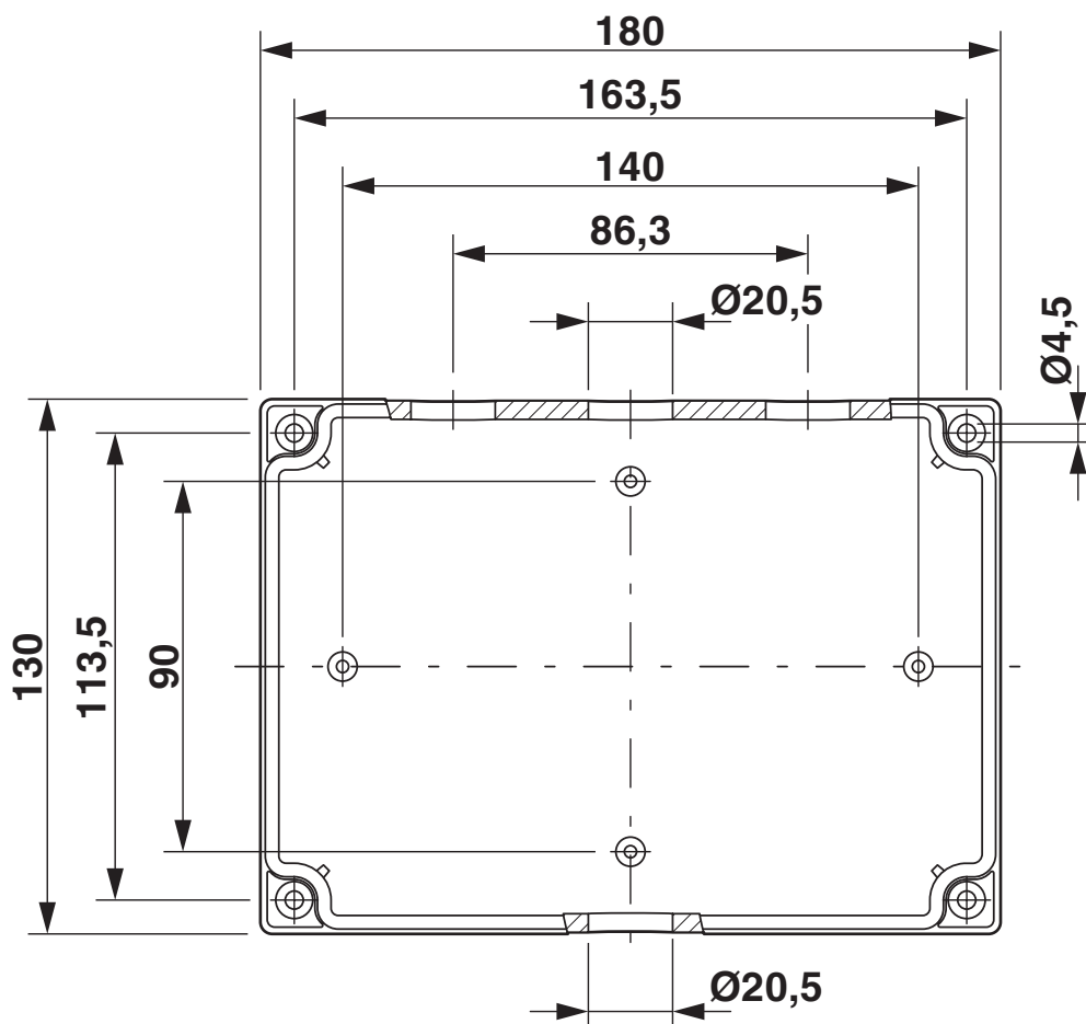
Rysunek wymiarowy
