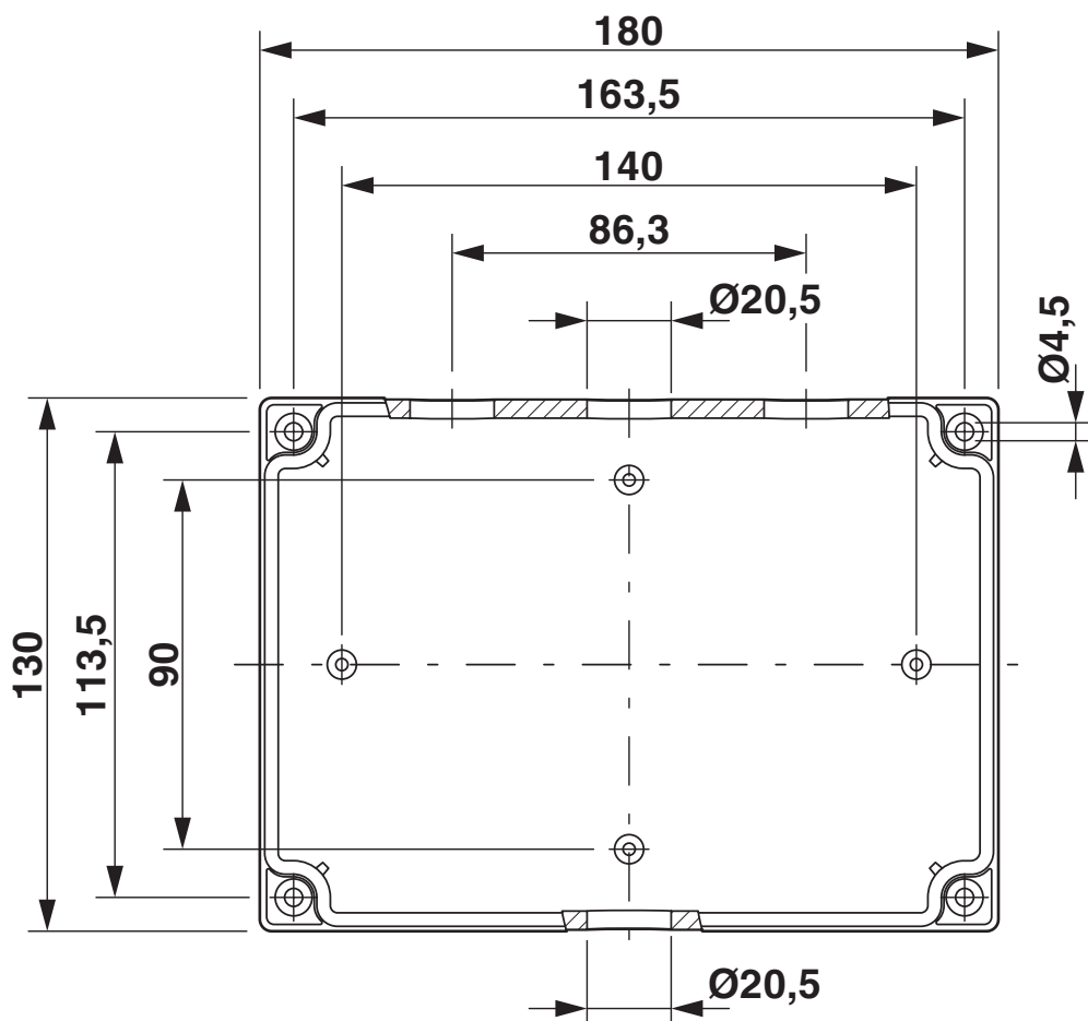
Rysunek wymiarowy
