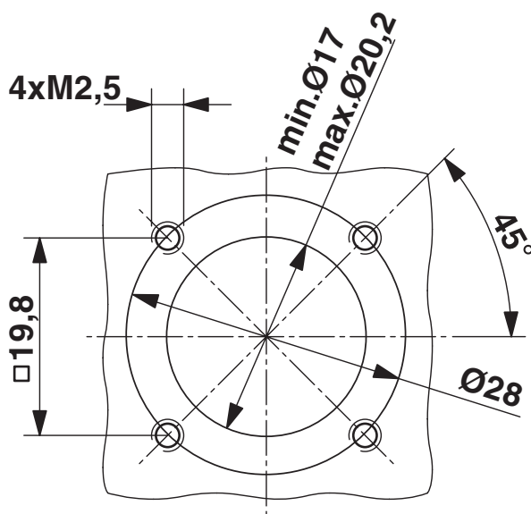
Rysunek wymiarowy
