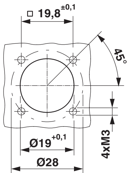
Rysunek schematyczny
