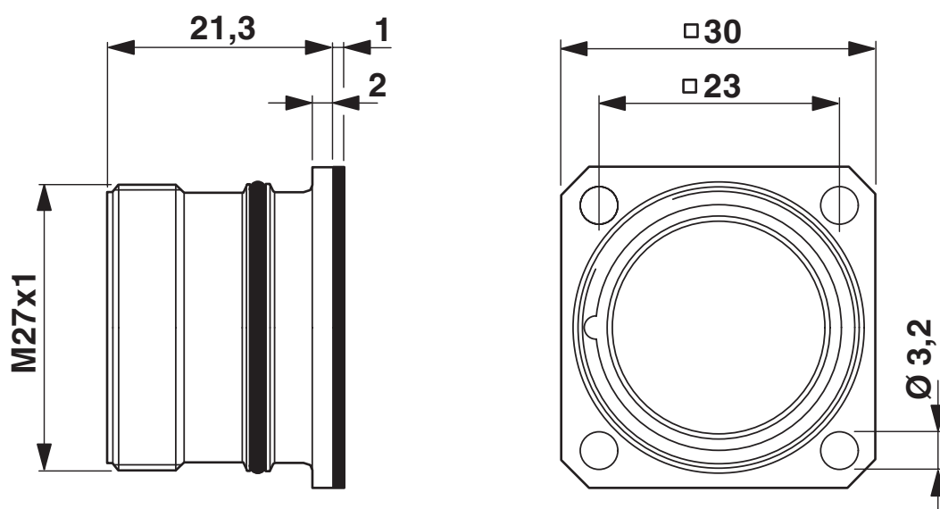
Rysunek wymiarowy
