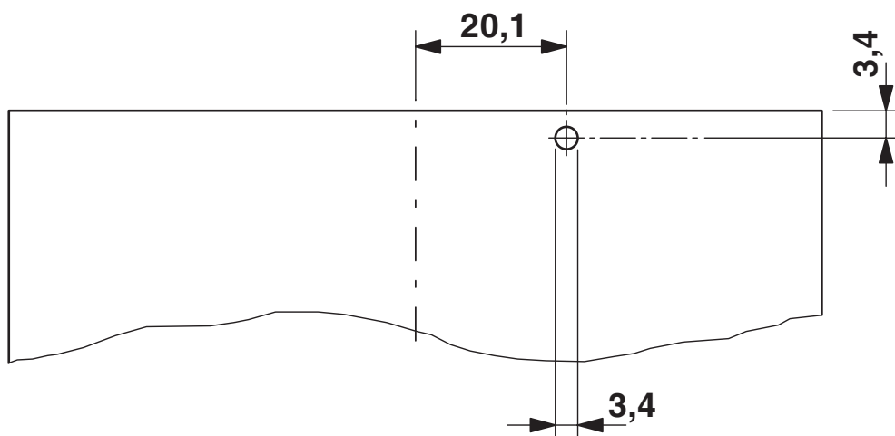
Otworowanie/geometria płytek lutowniczych
