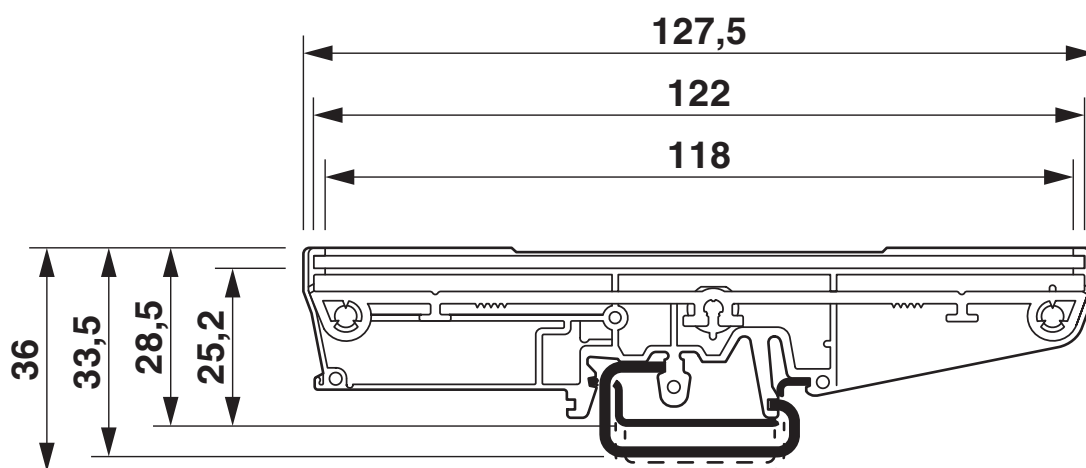
Rysunek wymiarowy
