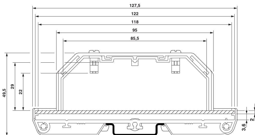
Rysunek wymiarowy
