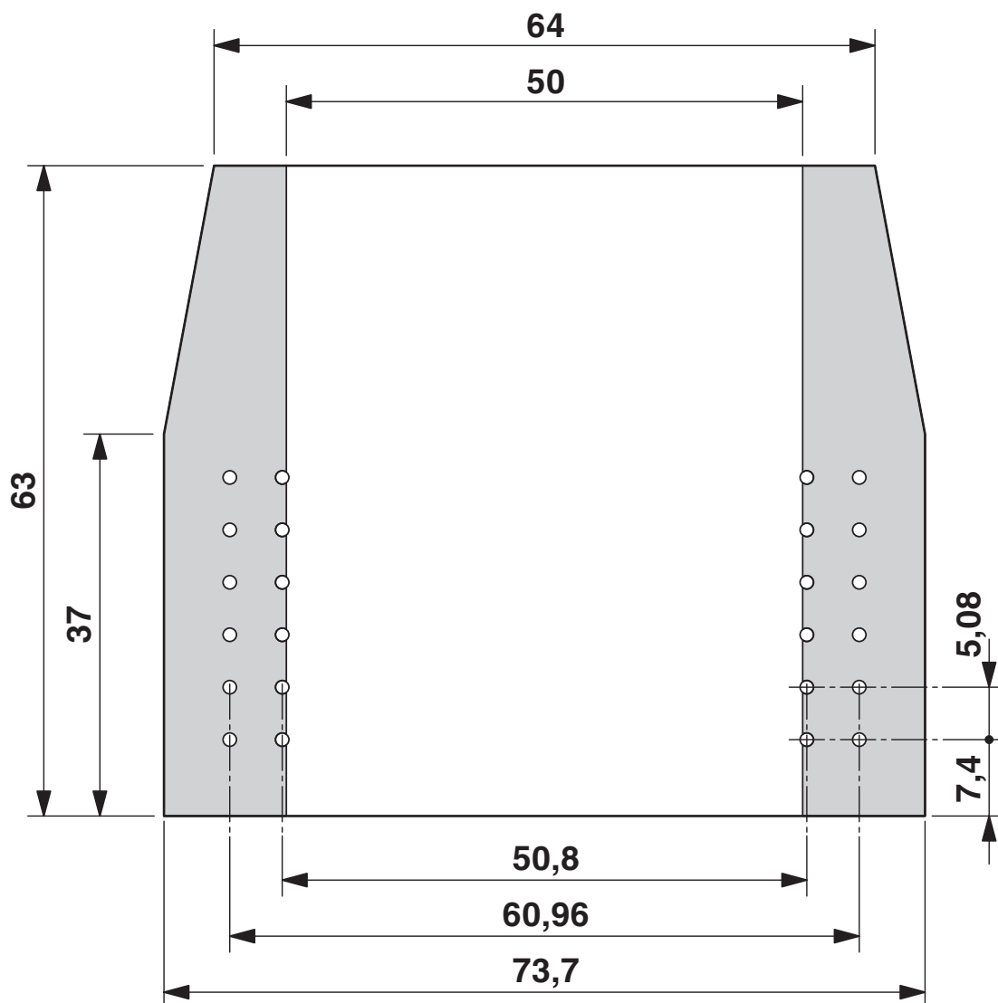
Rysunek wymiarowy
