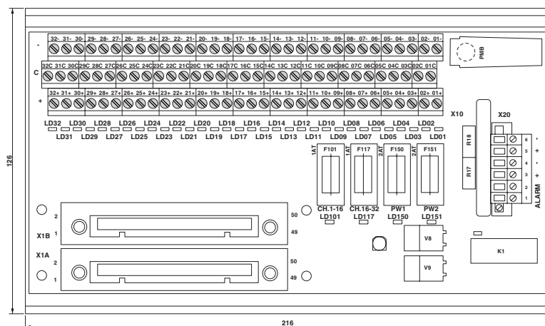
Rysunek wymiarowy
