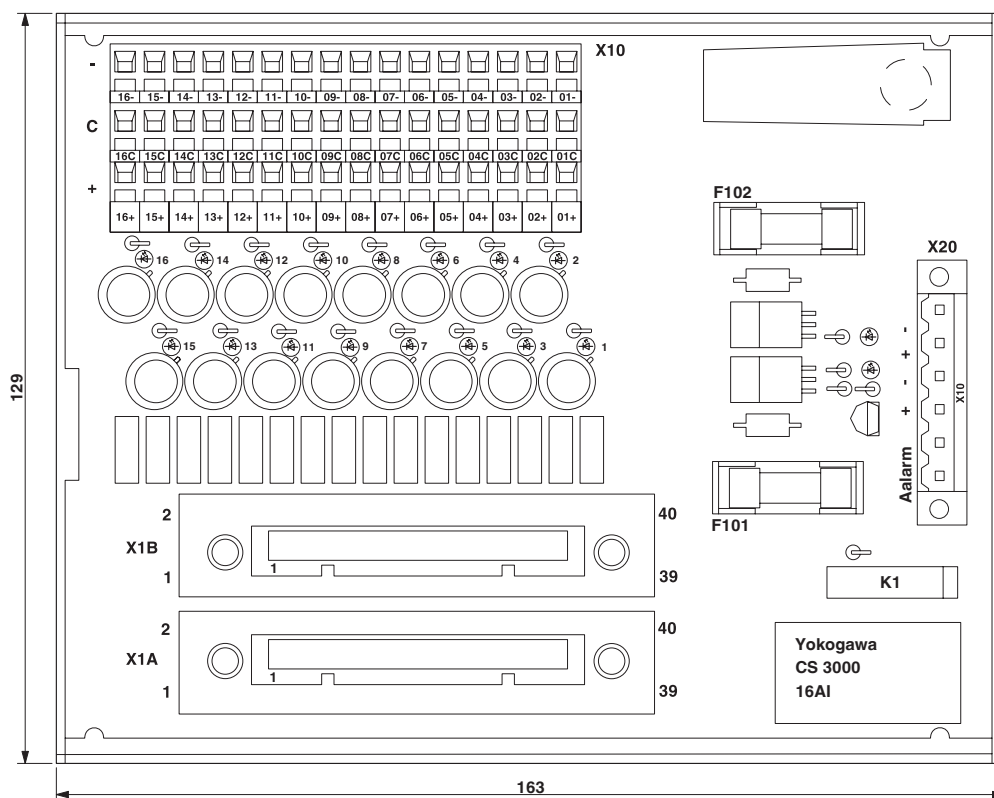
Rysunek wymiarowy
