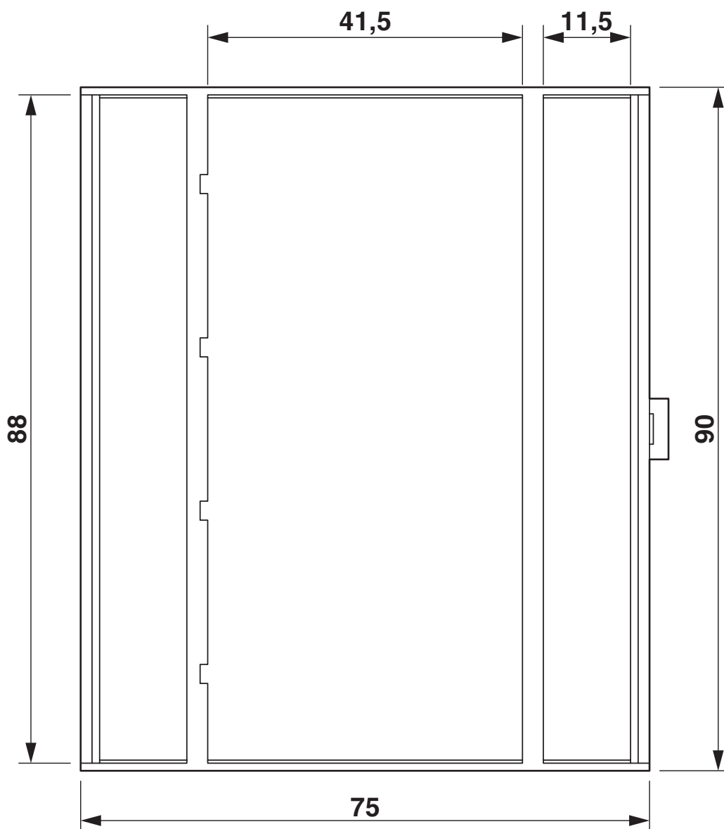
Rysunek wymiarowy
