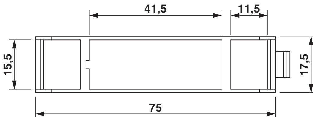
Rysunek wymiarowy
