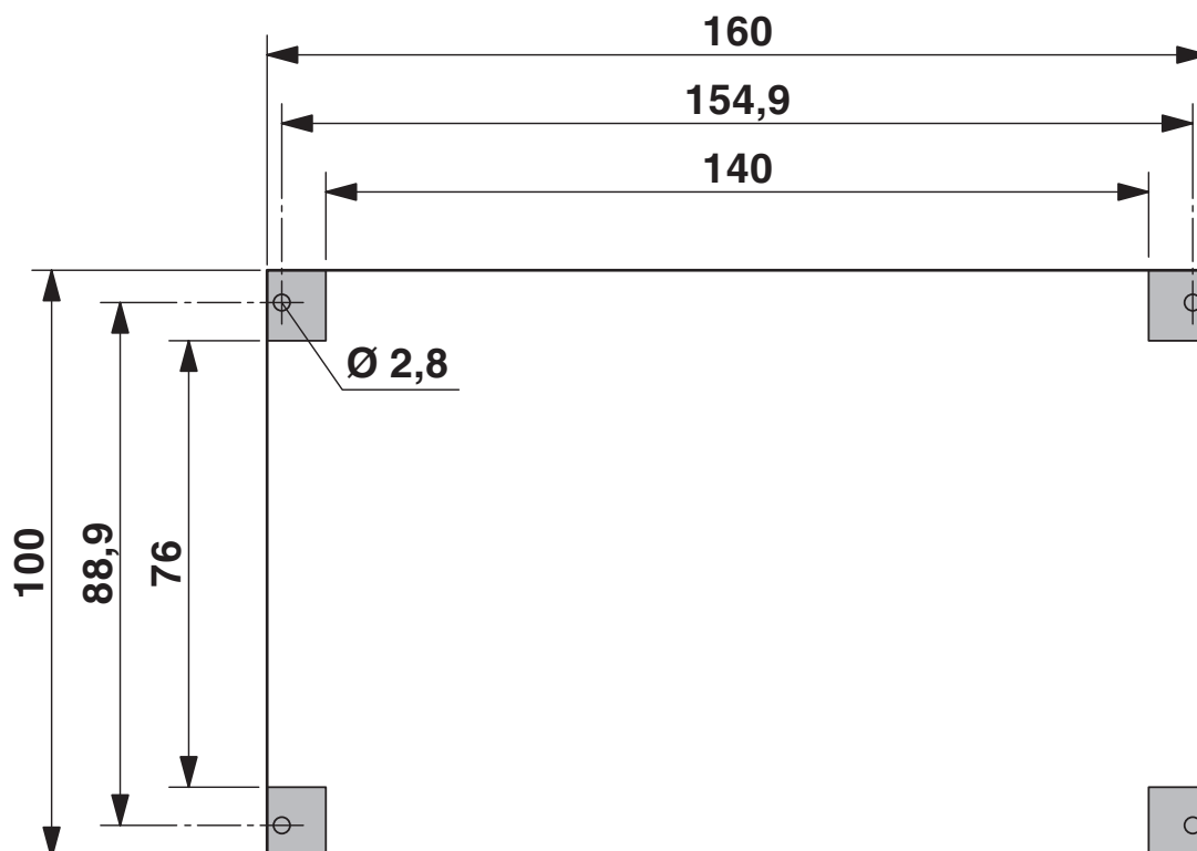
Rysunek wymiarowy
