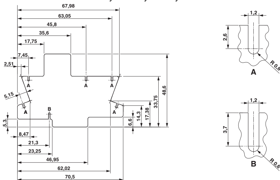
Rysunek wymiarowy
