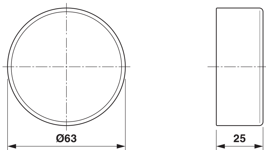
Rysunek wymiarowy
