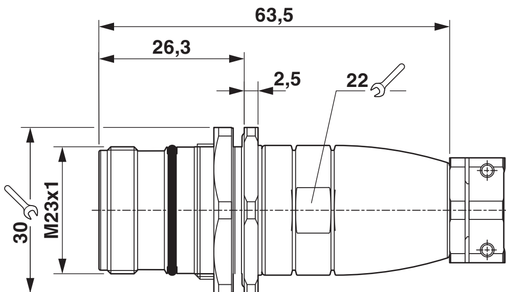
Rysunek wymiarowy
