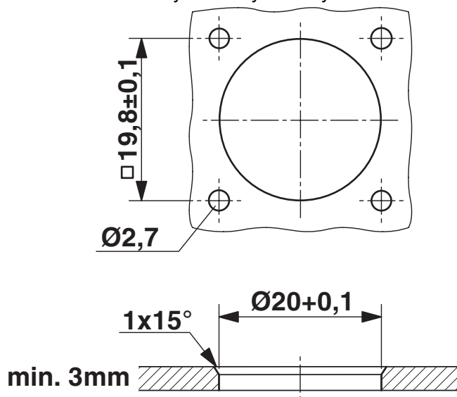
Rysunek wymiarowy
