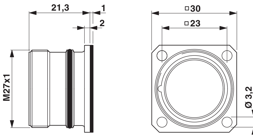
Rysunek wymiarowy
