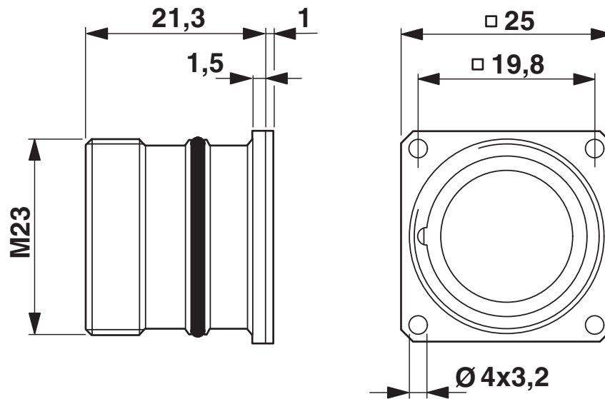
Rysunek wymiarowy
