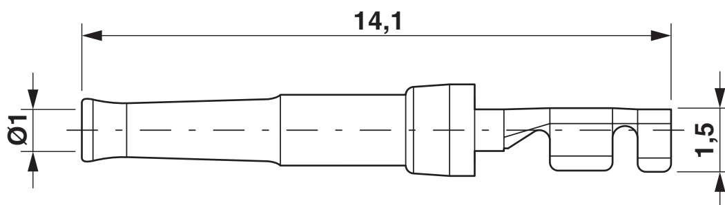
Rysunek wymiarowy
