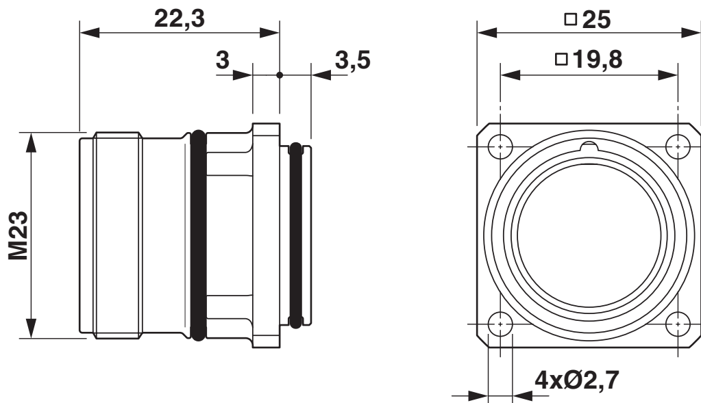
Rysunek wymiarowy
