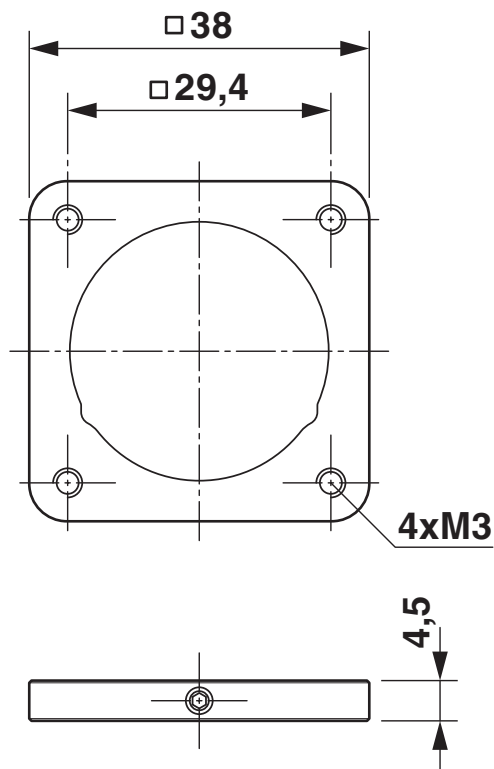
Rysunek wymiarowy
