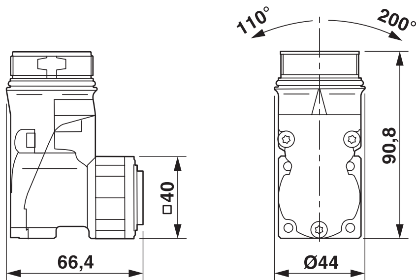
Rysunek wymiarowy
