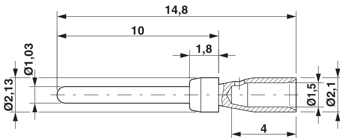
Rysunek wymiarowy
