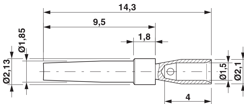
Rysunek wymiarowy
