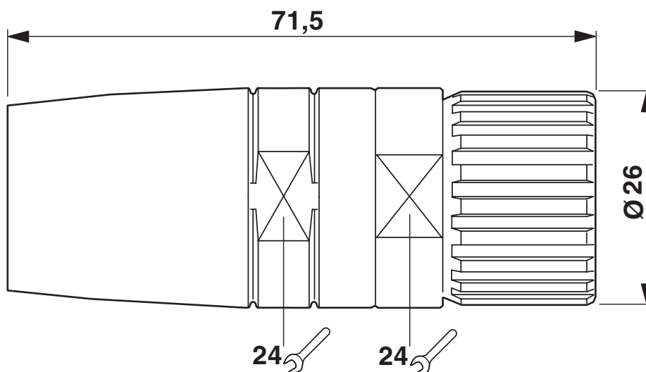
Rysunek wymiarowy
