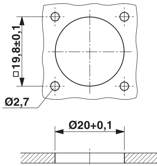
Rysunek wymiarowy
