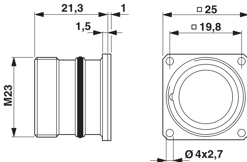
Rysunek wymiarowy
