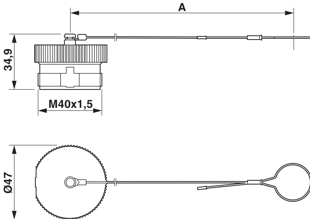
Rysunek wymiarowy
