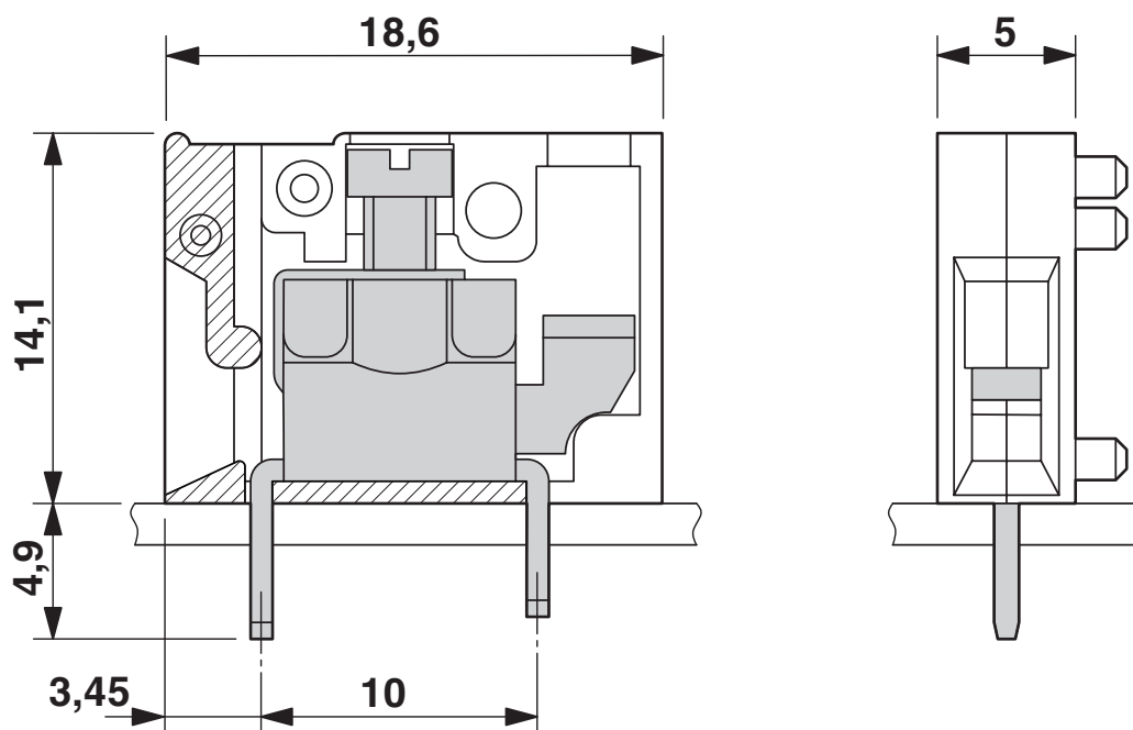
Rysunek wymiarowy
