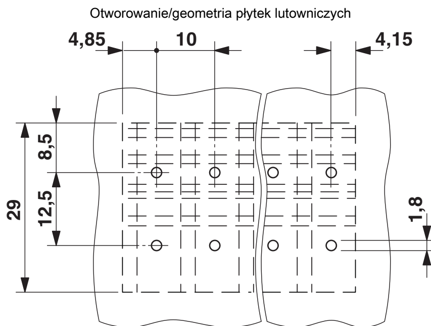
Rysunek wymiarowy
