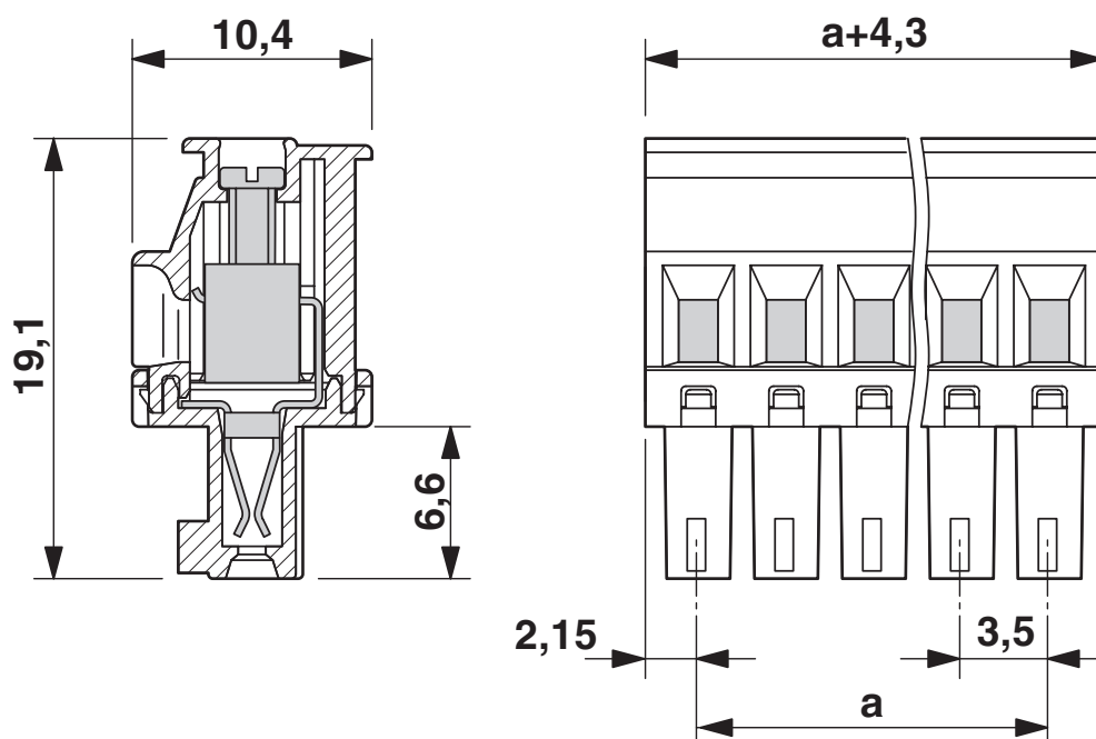
Rysunek wymiarowy
