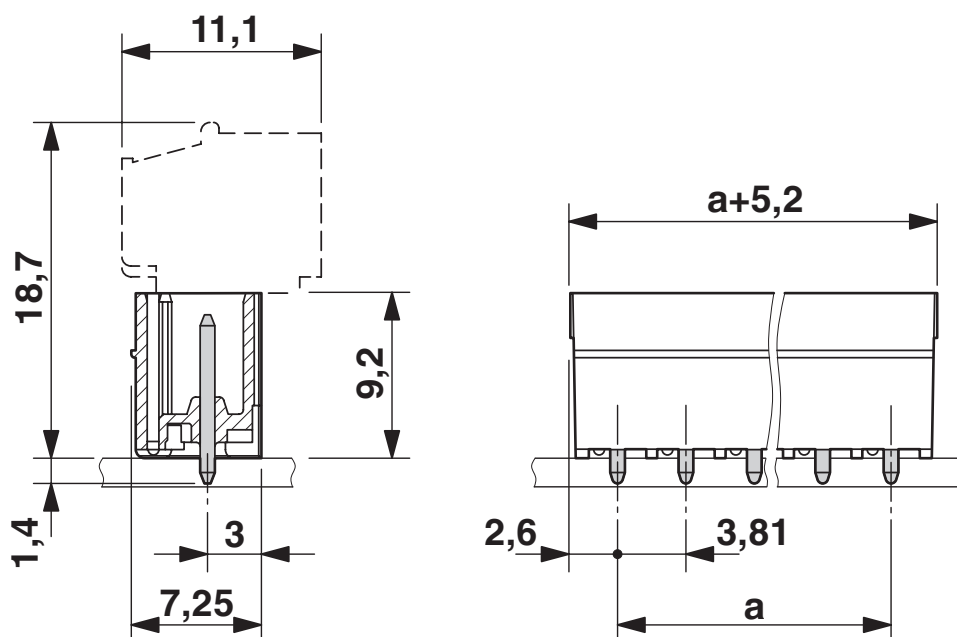
Rysunek wymiarowy
