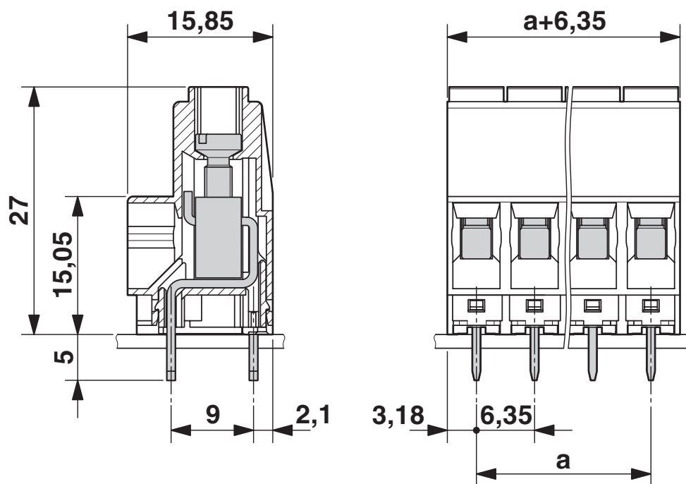
Rysunek wymiarowy
